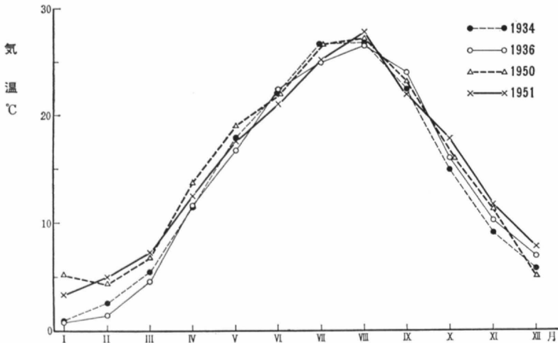
図1 京都市における調査各年の各月平均気温
