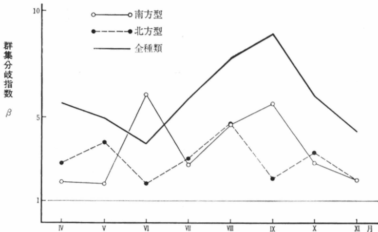
図 5 各月の群集分岐指数値
